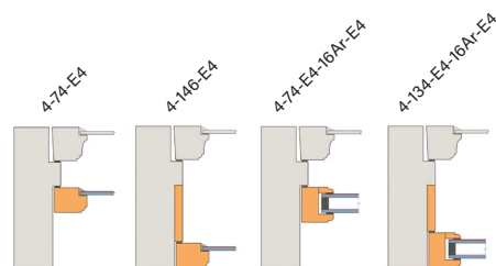
Varevinduer - varianter (SINTEF, Homb & Uvsløkk 2012)
